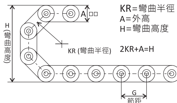
圖二：彎曲高度算式圖
