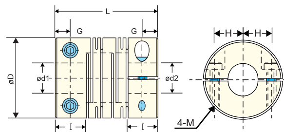
外徑Ø40~Ø63
