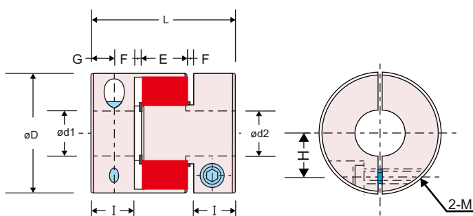
外徑 \phi 20~ \phi 30
