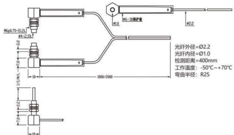
BT6YTZ-T□-1M/2M (凸管長度)
