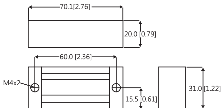
磁力鎖本體
