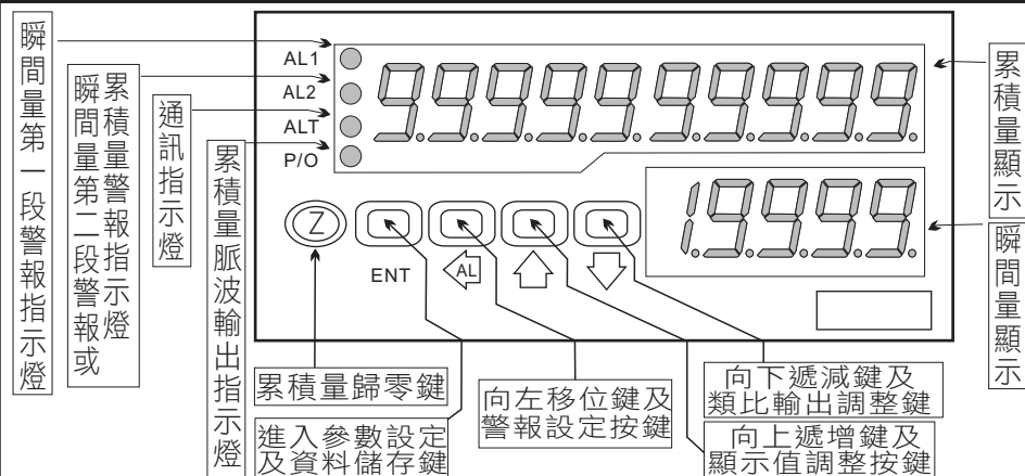
顯示面板指示燈及操作按鍵說明圖
