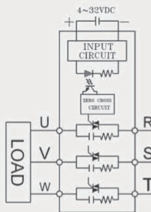
TSR-25DA-□ / TSR-40DA-□
