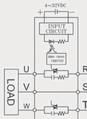
TSR-50DA-□ / TSR-75DA-□
