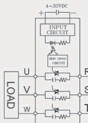
TSR-25DA-□ / TSR-40DA-□
